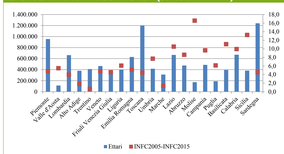
Figura 2: Stime preliminari delle superfici forestali nelle regioni italiane e variazioni % tra inventari (stime CREA-MPF)
